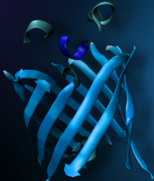
Proteína 1EMA (VMD)
