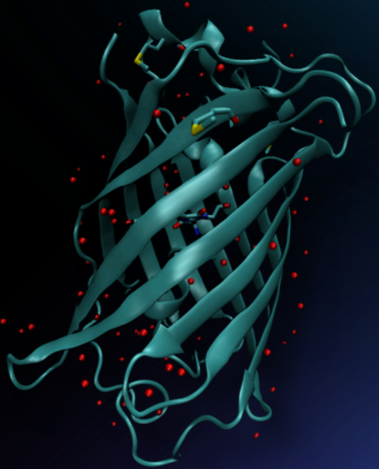
Constituintes da proteína: 95 moléculas de água
